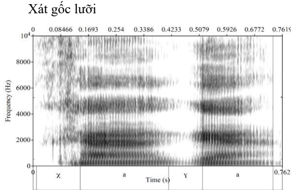
Hình 13. Ảnh phổ của phụ âm [χ] trong từ kha, [γ] trong từ ga.
