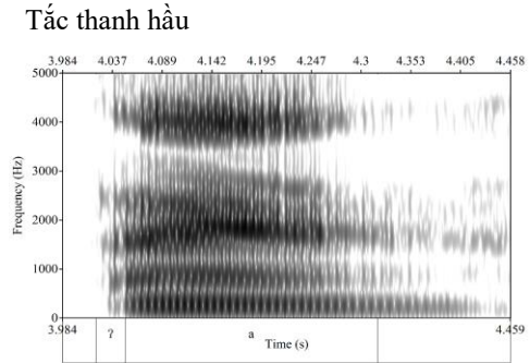
Hình 9. Ảnh phổ của phụ âm [ʔ] trong từ a
