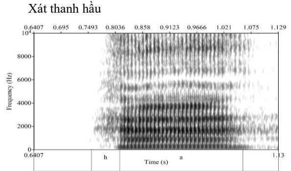
Hình 14. Ảnh phổ của phụ âm [h] trong từ ha. Âm [h] có vệt phổ rất yếu (Hình 14).
